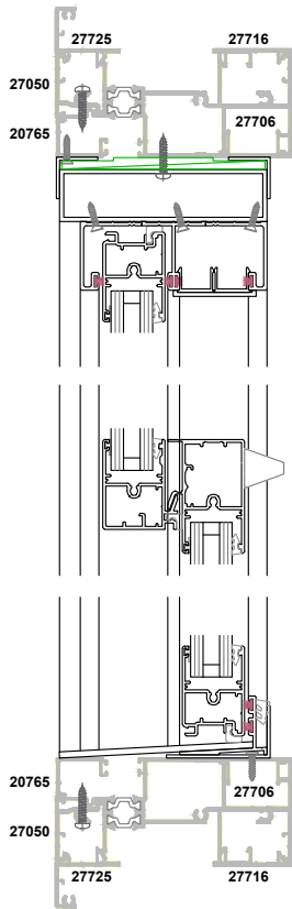
Section A:A
