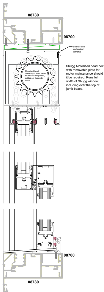
Section A:A
