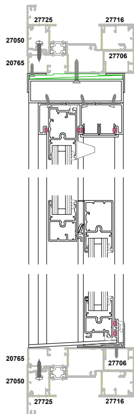
Section A:A
